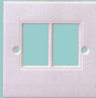
1021 - 2 Port Module - 22 x 37 mm
